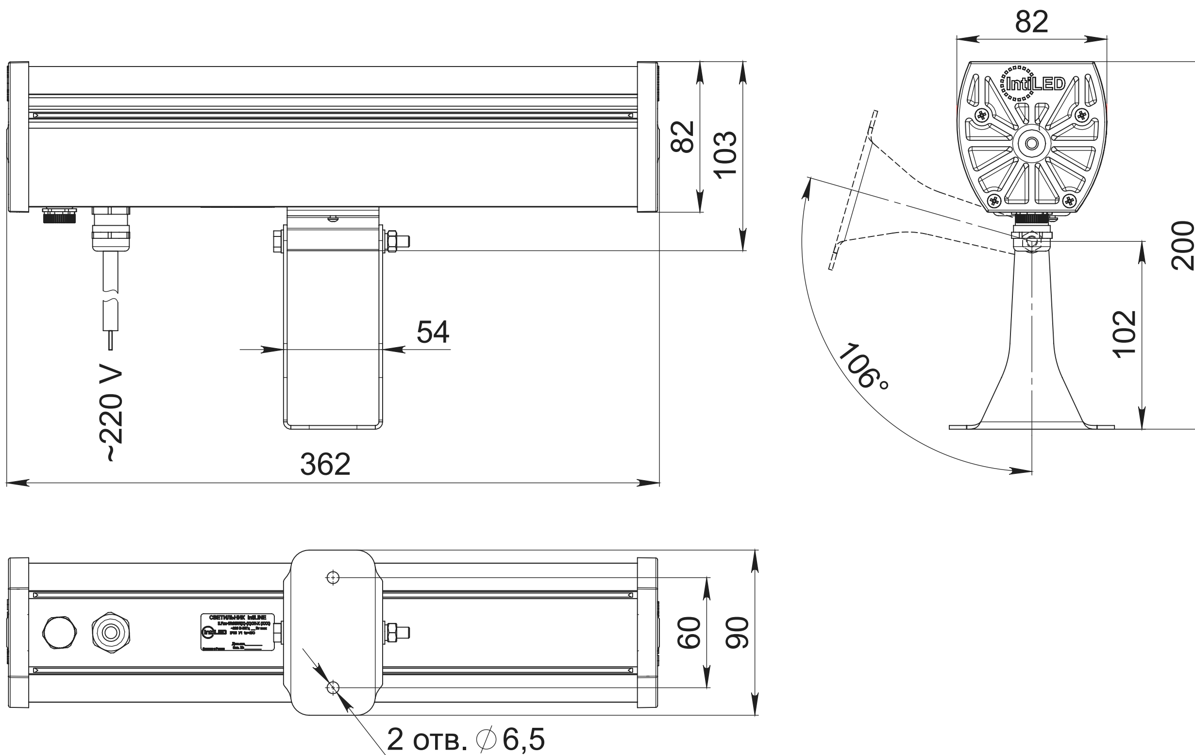
Габаритный чертеж монохромных светильников серии IntiLINE (условная длина 30)
