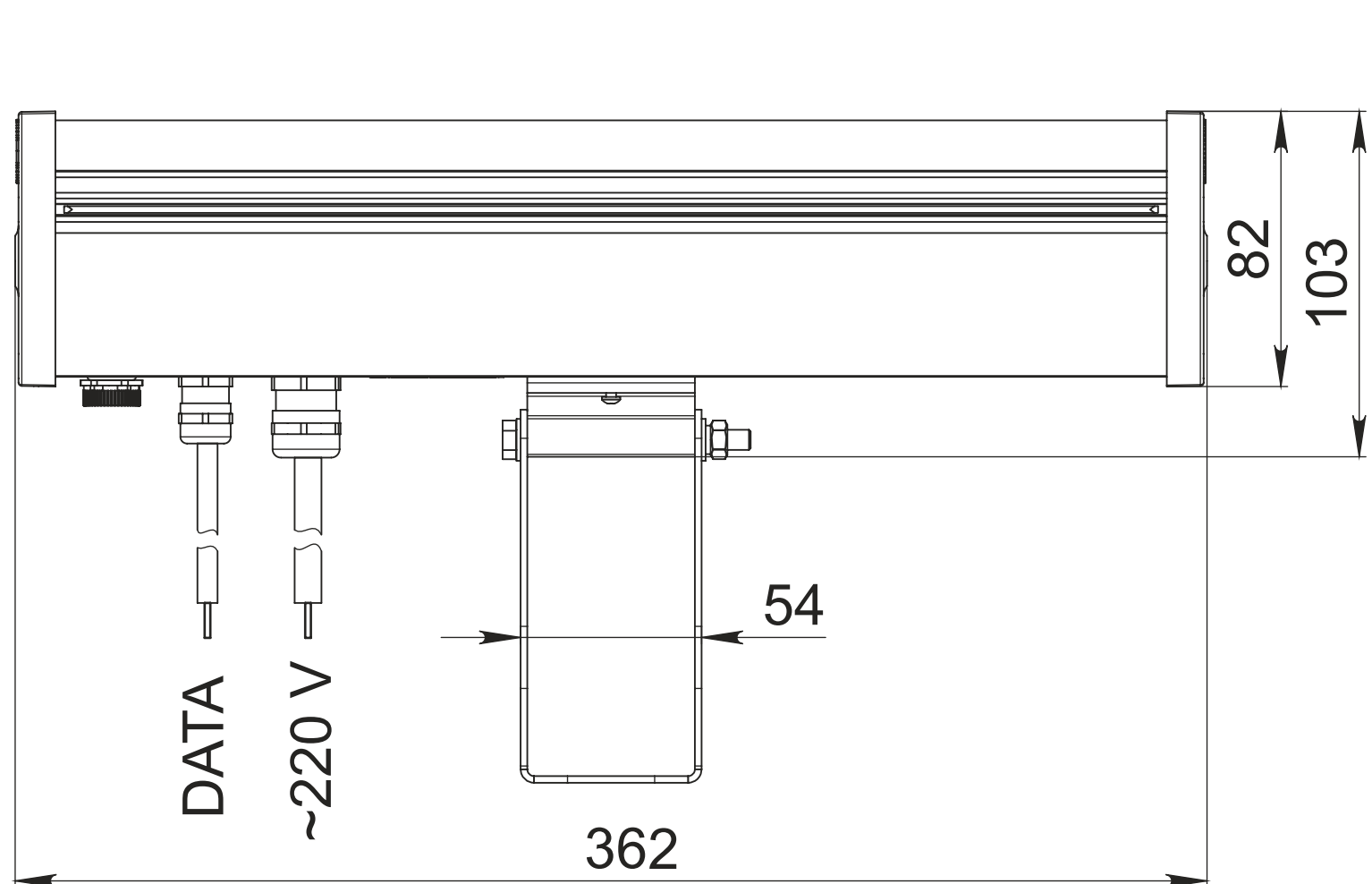
Габаритный чертеж цветодинамических светильников серии IntiLINE (условная длина 30)
