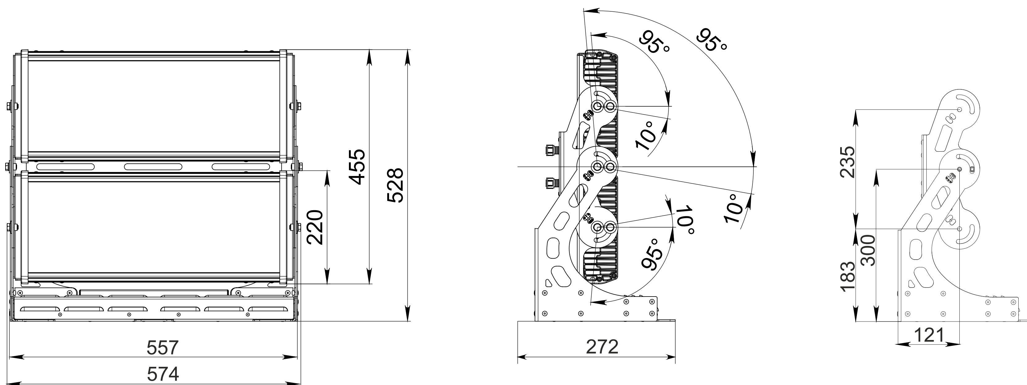
Габаритный чертеж цветодинамических светильников серии IntiSTARK big-block
