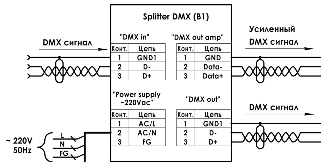
Усиление с разветвлением
