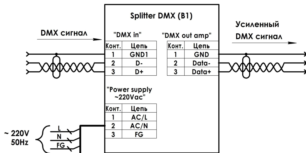
Усиление без разветвления
